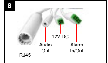
Anschluss-Stecker für die Kamera
